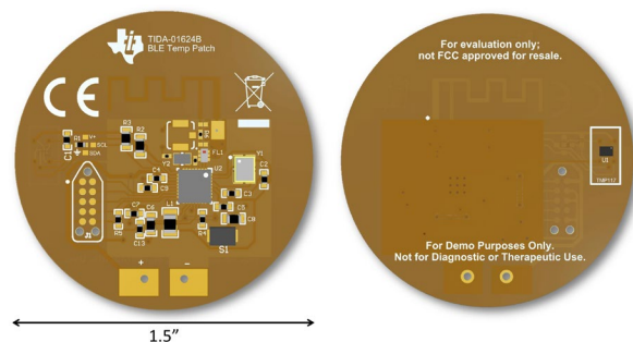
Abbildung 5. PCB-Pflaster-Referenzdesign.
