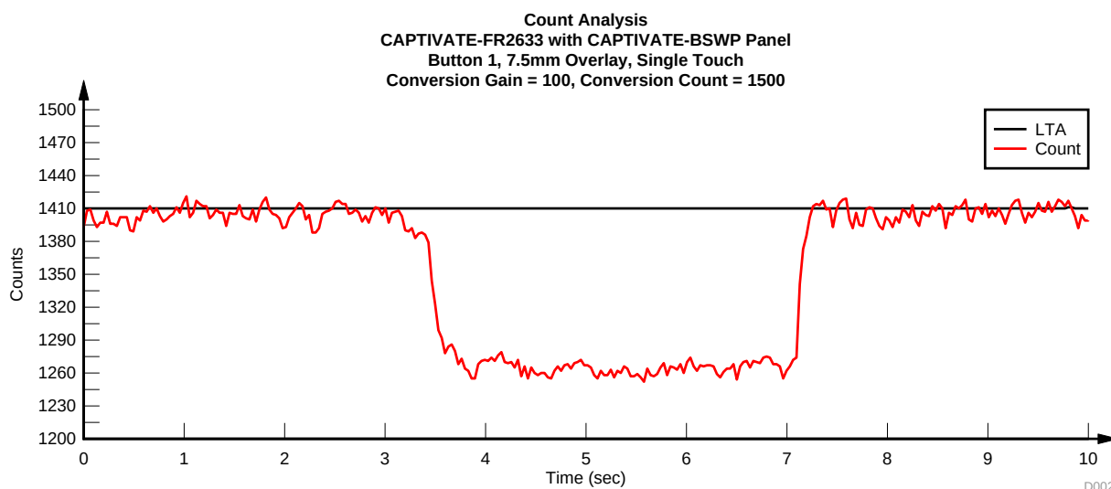
图 10. 使用 7.5 mm 镀层时的计数分析
