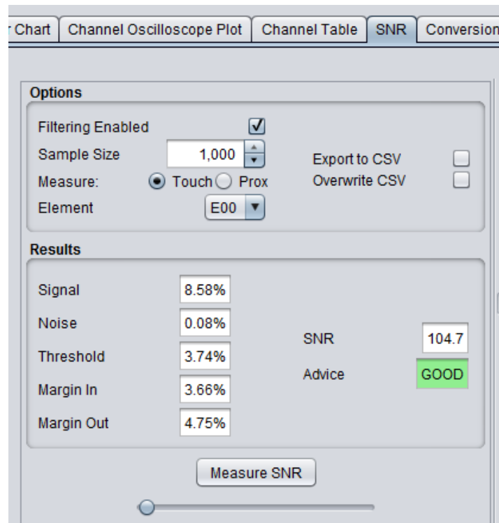
图 3. 执行测试后的 SNR 视图
