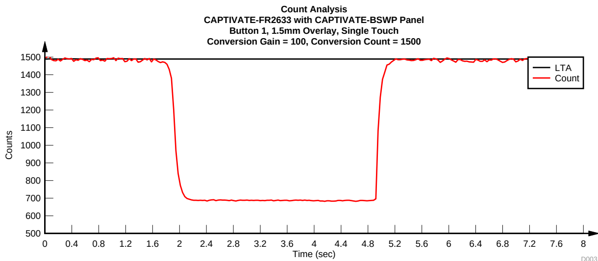
图 12. 使用 1.5 mm 镀层时的计数分析
