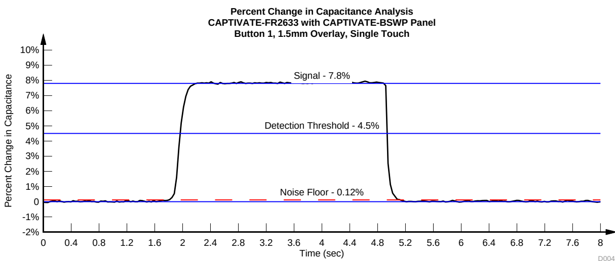
图 13. 使用 1.5 mm 镀层时的变化百分比分析
