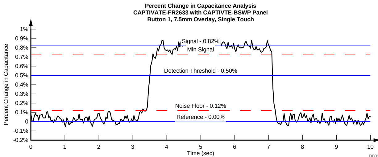
图 11. 使用 7.5 mm 镀层时的变化百分比分析
