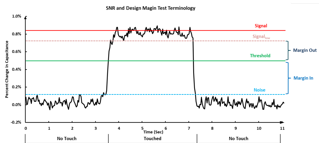
图 8. 设计裕度术语
