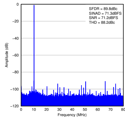
图 7-7. FFT for 170-MHz Input Signal
