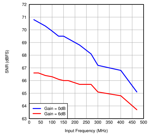
图 7-93. SNR vs Input Frequency (CMOS)
