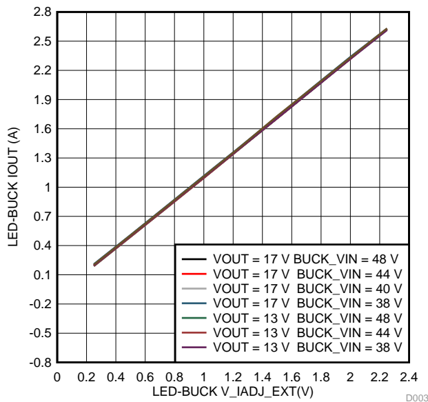
图 52. IOU vs V_IADJ_EXT
